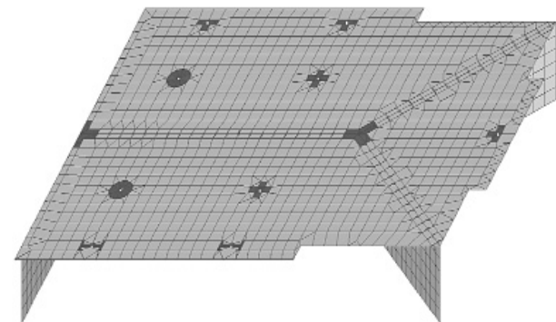
Рис. 8. Схема МКЭ перекрытия с генерацией АЖТ
